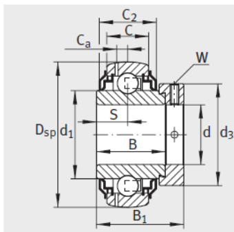
GE..-KRR-B-2C
