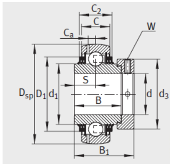
GE..-KTT-B
