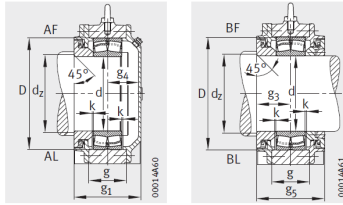
设计类型 A 带有 Taconite 密封的轴承座 适用于圆柱孔轴承 设计类型 B 带有迷宫密封的轴承座 适用于圆柱孔轴承
