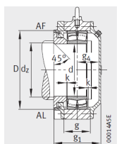
设计类型 A 带有迷宫密封的轴承座 适用于圆柱孔轴承
