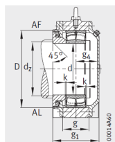
设计类型 A 带有 Taconite 密封的轴承座 适用于圆柱孔轴承
