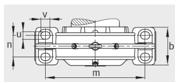
BND 轴承座的横截面, 适用于圆锥孔轴承: 见第 1441 页到第 1443 页
