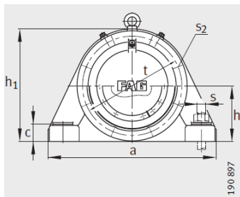
BND 轴承座的横截面, 适用于圆锥孔轴承: 见第 1441 页到第 1443 页
