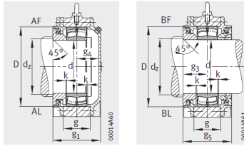
设计类型 A 带有 Taconite 密封的轴承座 适用于圆柱孔轴承
