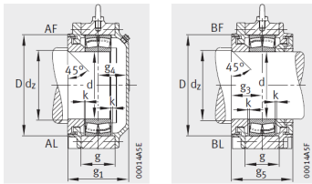
设计类型 A 带有迷宫密封的轴承座 适用于圆柱孔轴承
