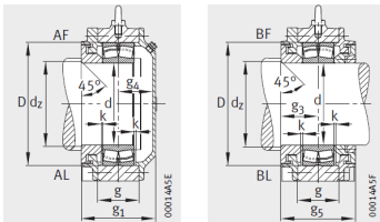
设计类型 A 带有迷宫密封的轴承座 适用于圆柱孔轴承 设计类型 B
