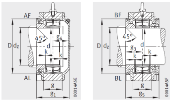
设计类型 A 带有迷宫密封的轴承座 适用于圆柱孔轴承 设计类型 B 带有 Taconite 密封的轴承座 适用于圆柱孔轴承
